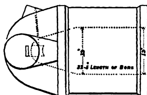
FIG. 22.—13-inch Mortar.
