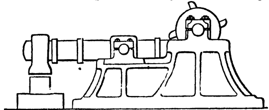
FIG. 3.—Tilt Hammer.
